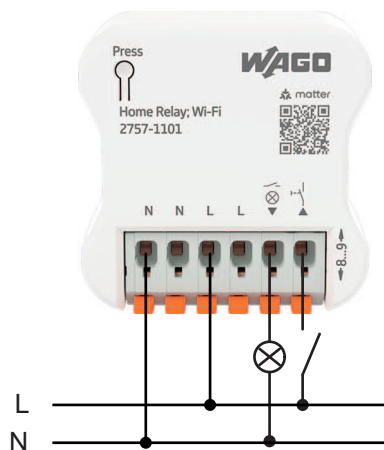
Abbildung 11: Anschlussbeispiel 1
