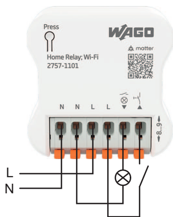
Abbildung 12: Anschlussbeispiel 2
