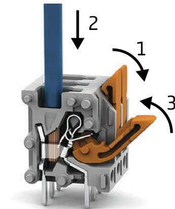
Abbildung 14: Feindrängige Leiter ohne Aderendhülse anschließen
